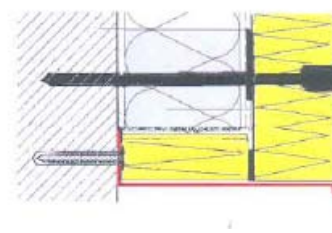
Figure 2c : Ancien profilé disqué Nouveau profilé standard
