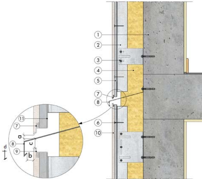
Figure 13 - Compartimentage horizontal de la lame d'air
