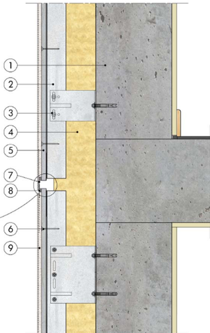
Figure B1 – Fractionnement au droit de chaque plancher
