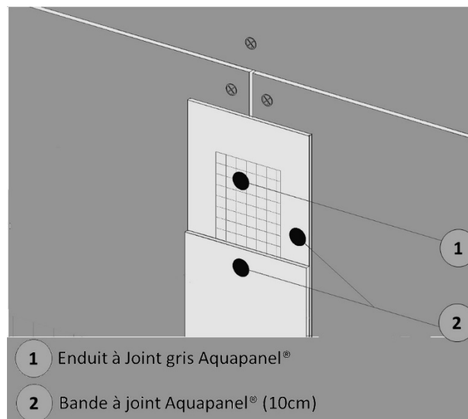
Figure 6bis - Jointoiment - Mise en œuvre des joints entre plaques – détails
