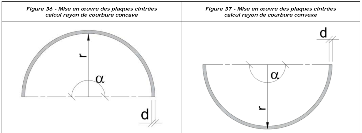
Figure 38 - Mise en œuvre des plaques cintrées – Exemple de gabarit pour pré-cintrage des plaques AQUAPANEL®
