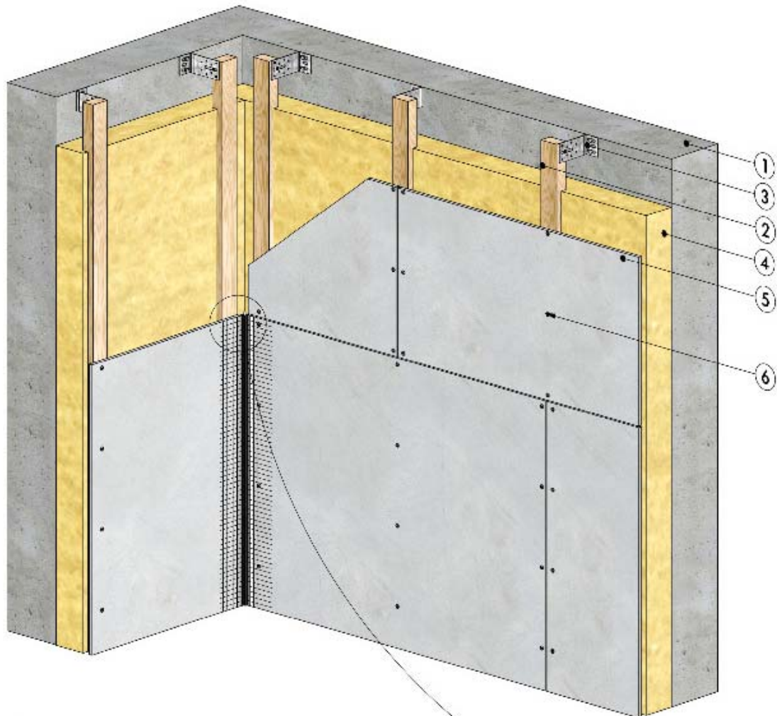
Figure 10 - Angle rentrant - fractionnement dans l'angle
