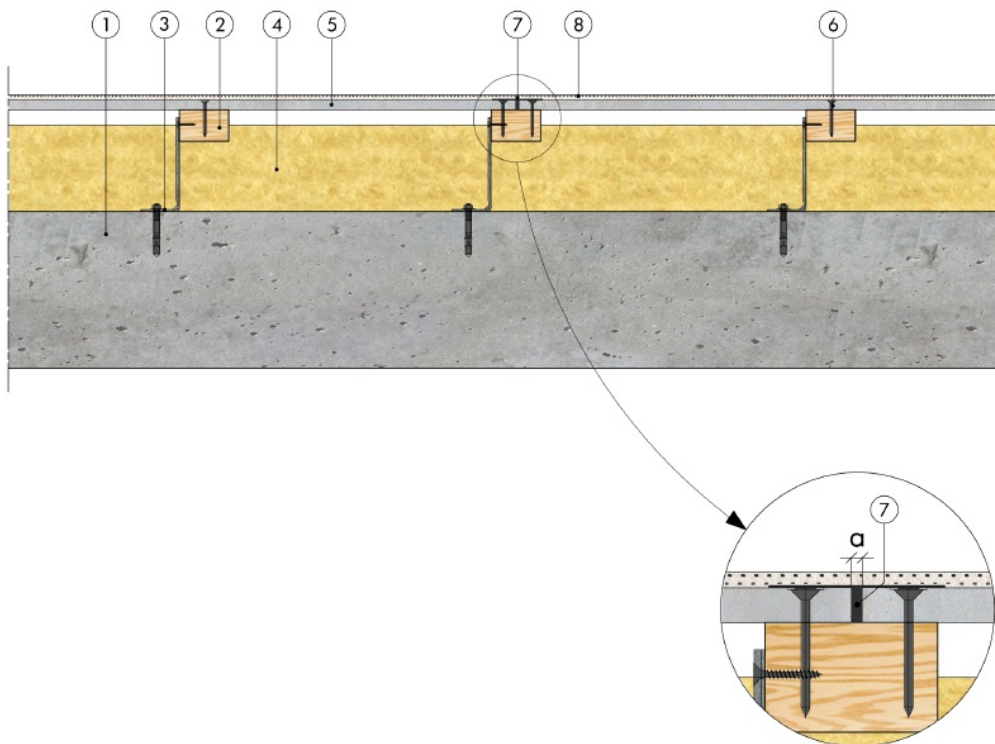
Figure 6 - Jointoiment - Mise en œuvre des joints entre plaques – Coupe horizontale
